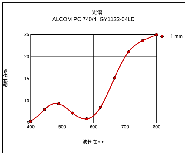
光谱
